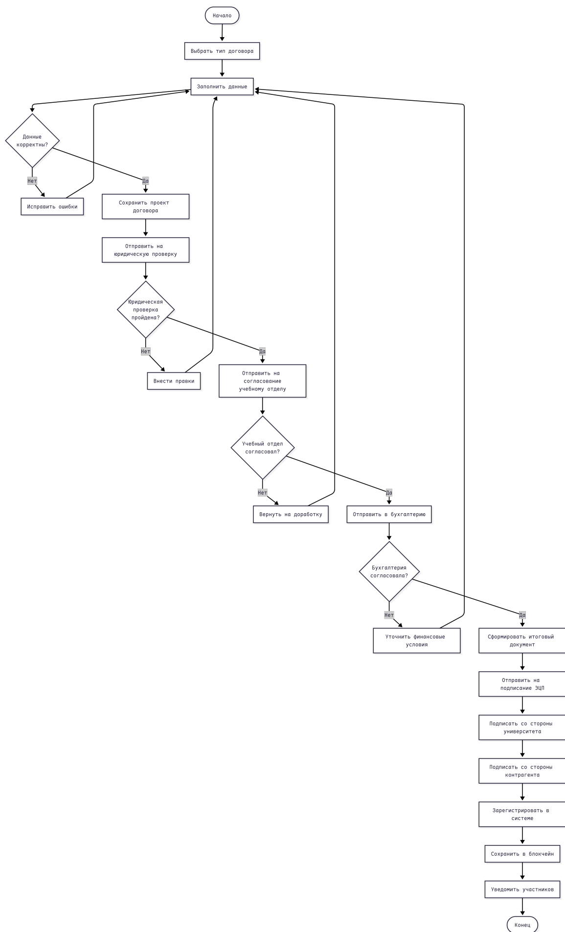
Рисунок 1.2 — Диаграмма активности: создание и согласование договора
