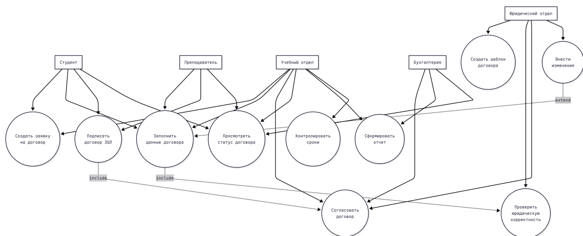
Рисунок 1.1 — Диаграмма прецедентов системы SmartContracts
