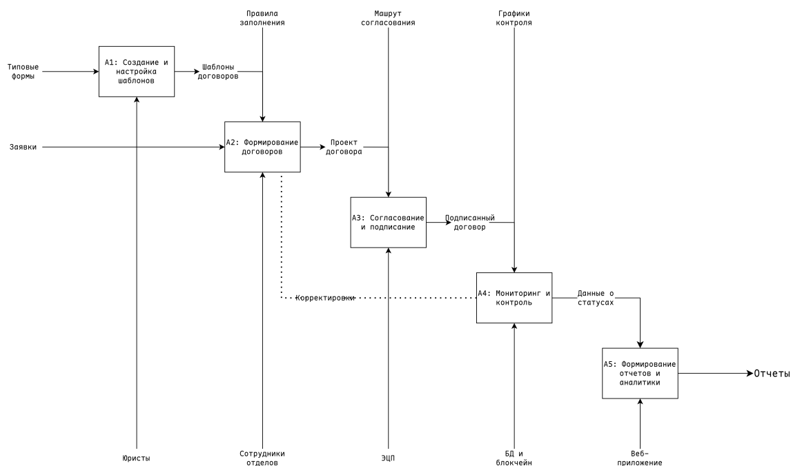
Рисунок 1.3 — IDEF0: Контекстная диаграмма A-0
