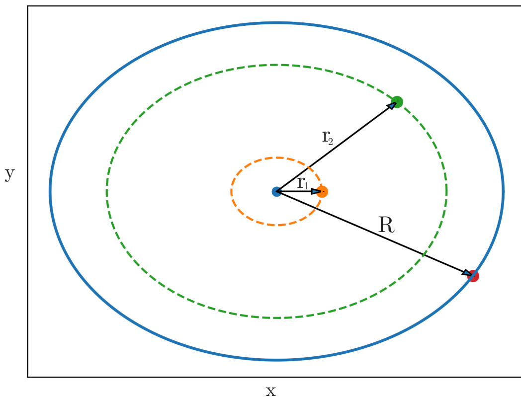
Рис. 3: Шар.
